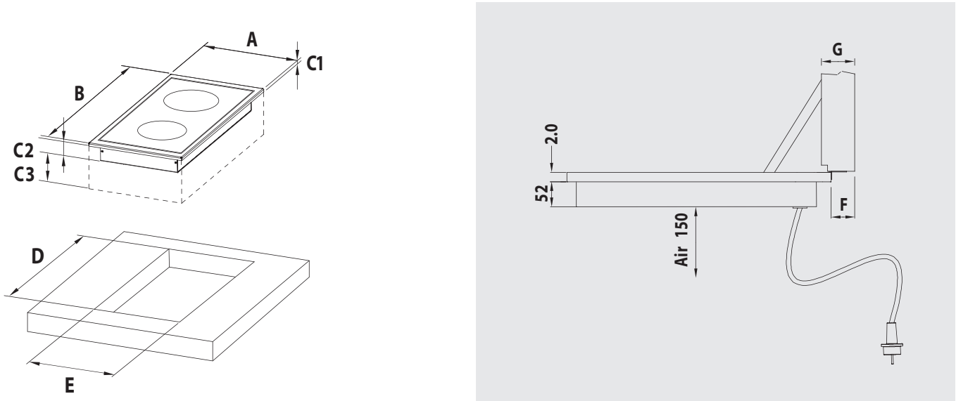
DISEGNO TECNICO 5
