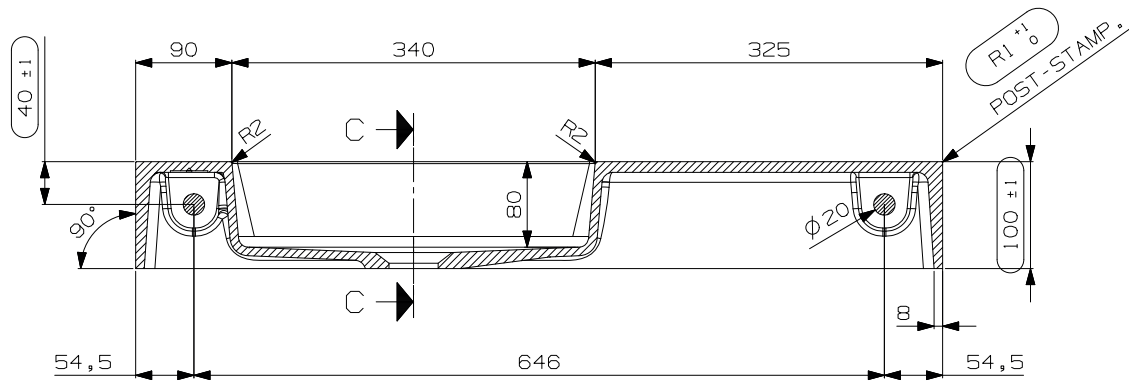
SECTION A-A SCALE 1:5
